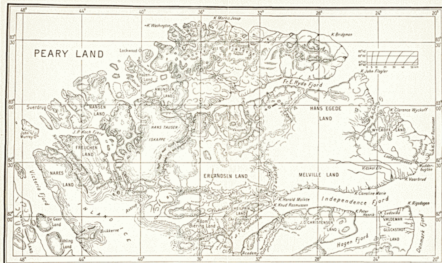
Fig. 11. Hele Pearyland med skitsemæssigt påførte ændringer fra Lauge Koch's originalkort: „Physiographical Map of Pearyland“ 1938. Medd. om Grønland, Bd. 130, nr. 1. (Færdigtegnet oktober 1950 og forevist som lysbillede for Det Kongelige Danske Geografiske Selskab og Det Grønlandske Selskab på fællesmødet den 9. november 1950).
