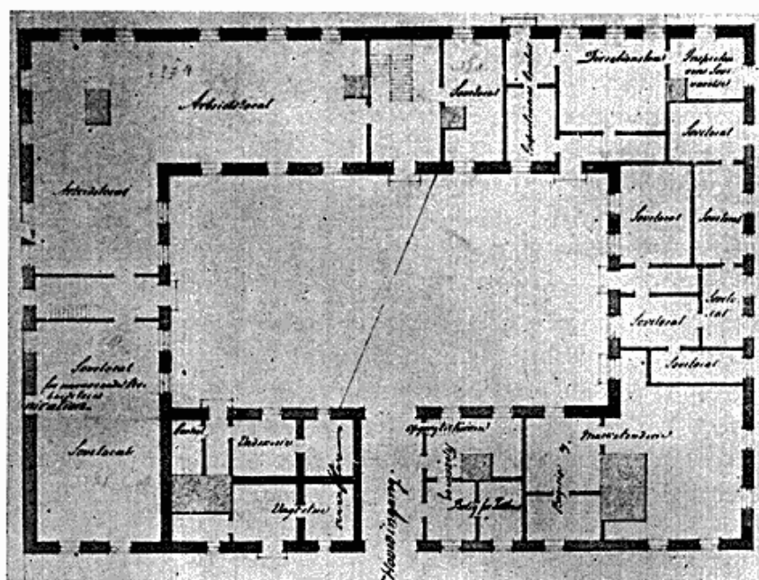
Plan af tugthuset stueetage, tegnet af Friis i 1843. (Rigsarkivet.)
