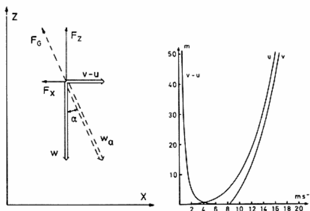
Fig. 1. The frictional resistance is directly opposite the relative velocity w_a , determined by the vertical velocity w and the relative horizontal velocity v-u of the drop. The horizontal component of the frictional resistance is called F_x , the vertical component F_z . Fig. 1. Modstanden mod en dråbes bevægelse er modsat rettet den relative hastighed w_a , bestemt ved vertikal faldhastighed w og relativ horisontal hastighed v-u . Gnidningsmodstandens horisontale og vertikale komponenter er henholdsvis F_x og F_z .
