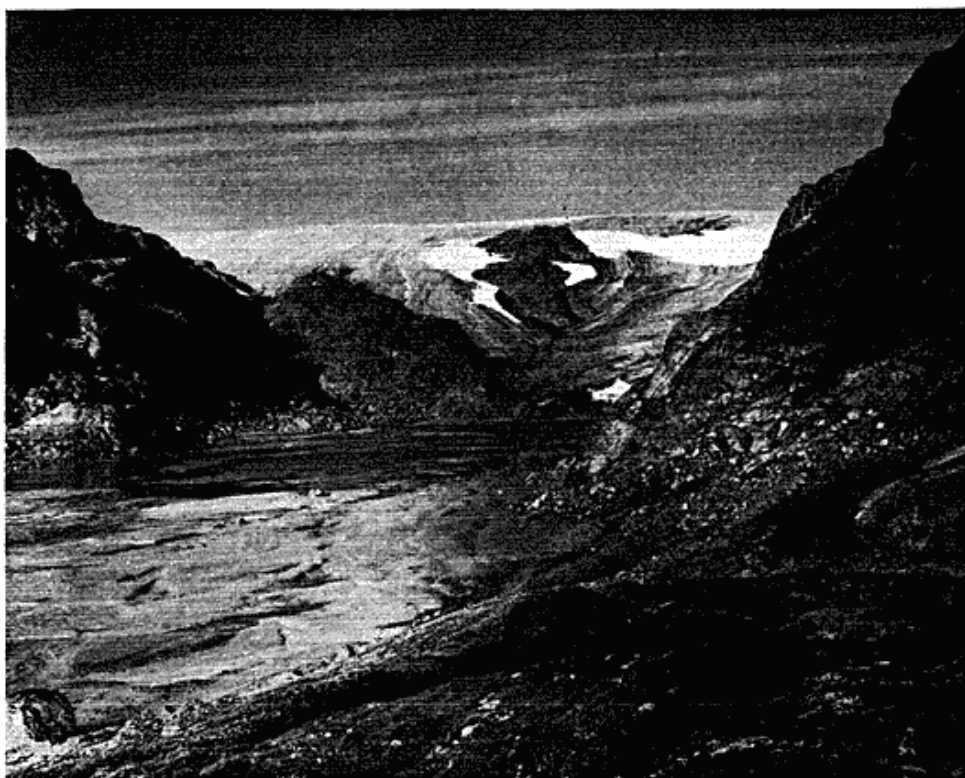
Fig. 2. Mitdluagkat Gletscheren 1958, fotograferet fra samme sted som i 1933. Fot. B. Fristrup.
