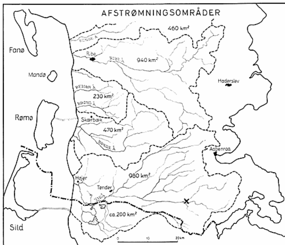
Fig. 1. Beliggenheden af nedbørsstation 09-420.
