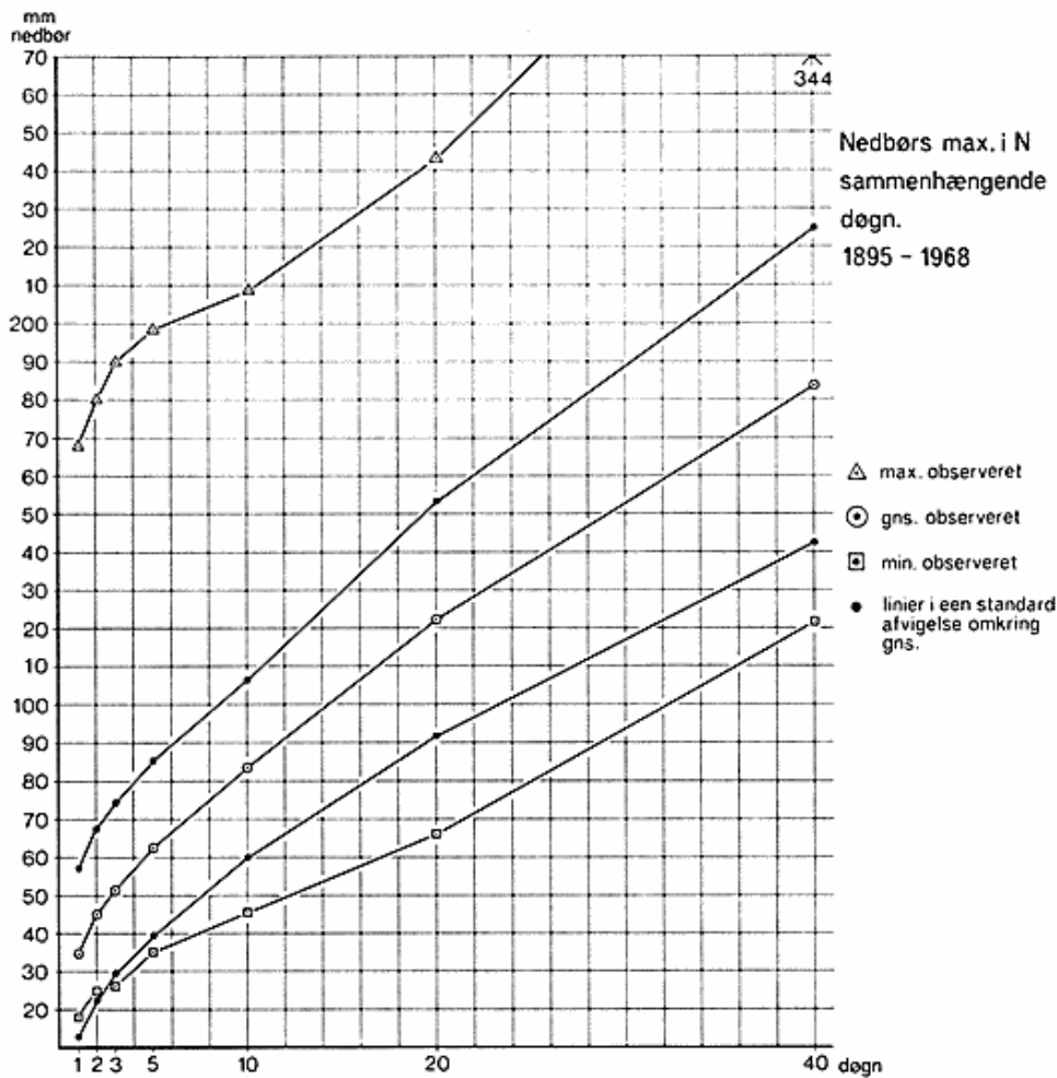
Fig. 2. Maksima i 1-40 døgn ud fra observerede værdier.
