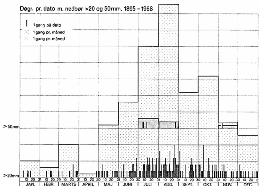
Fig. 8. Døgn i måleperioden 1895-1968 (÷ 1909-10), hvor nedbøren er større end 20 mm og 50 mm, afsat på den dato, hvor nedbøren er målt. Antallet af døgn er summeret pr. måned.
