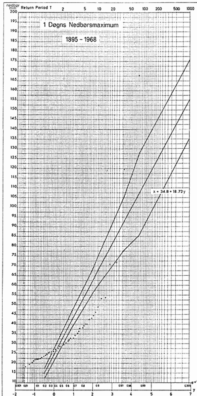
Fig. 5. 1-døgns årsmaksima. Gumbel plot. Ved store punkttætheder er punkter udeladt af tegnetekniske grunde.
