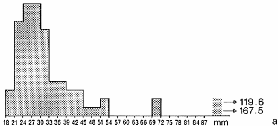
Fig. 4. Histogram over nedbørs-årsmaksima for 1, 3 samt 5 døgn.
