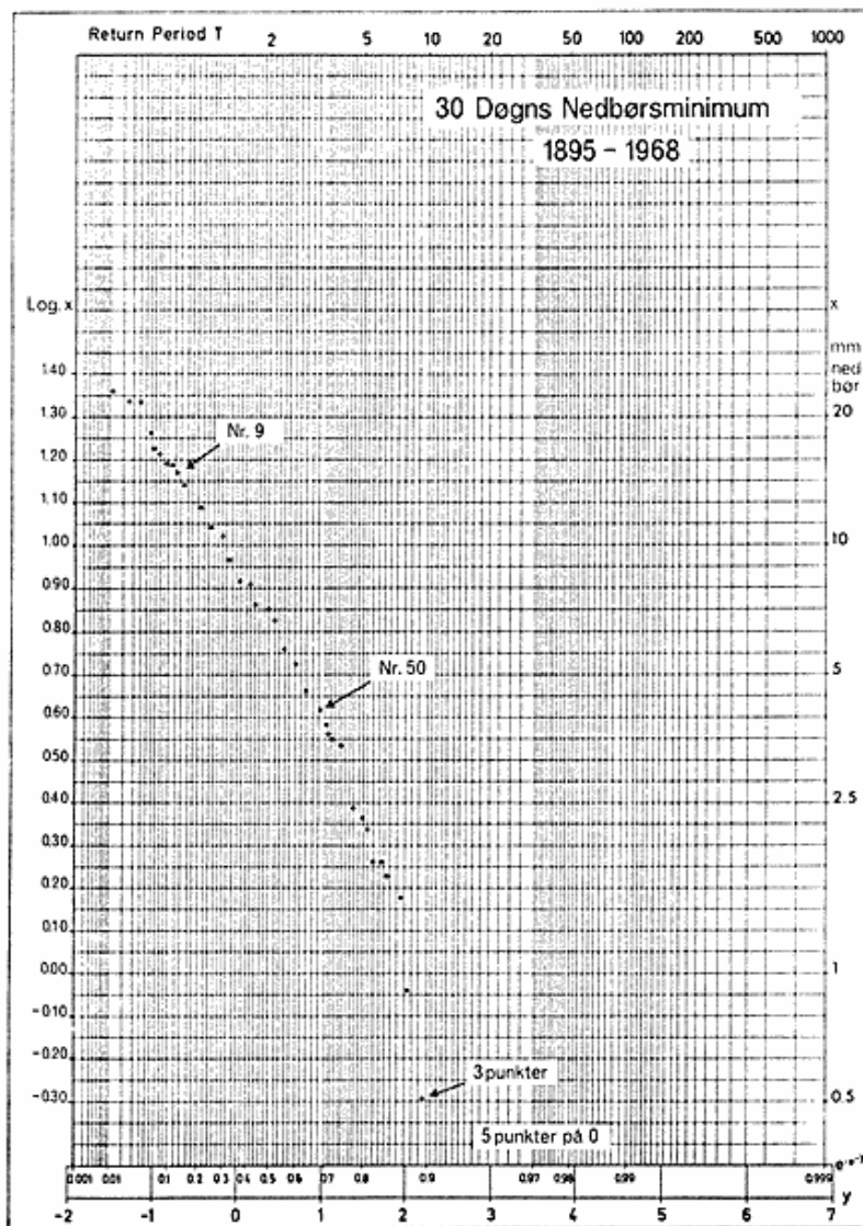
Fig. 11. 30-døgns årsminima. Gumbel plot. Punkter udeladt som i fig. 5.
