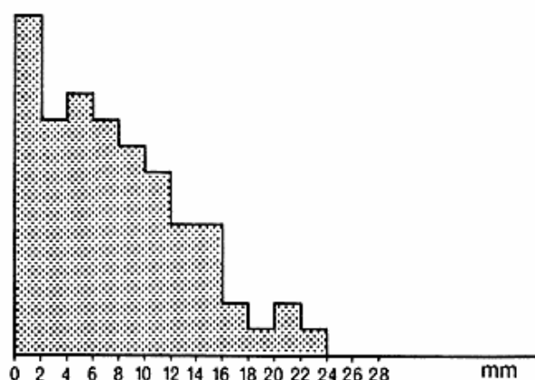
Fig. 12. Histogram over 30-døgns minima.
