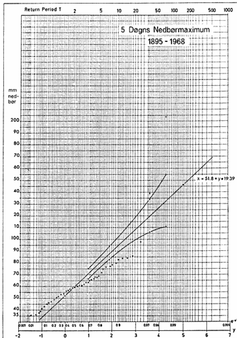
Fig. 7. 5-døgnns årsmaksima. Gumbel plot. Punkter udeladt som i fig. 5.
