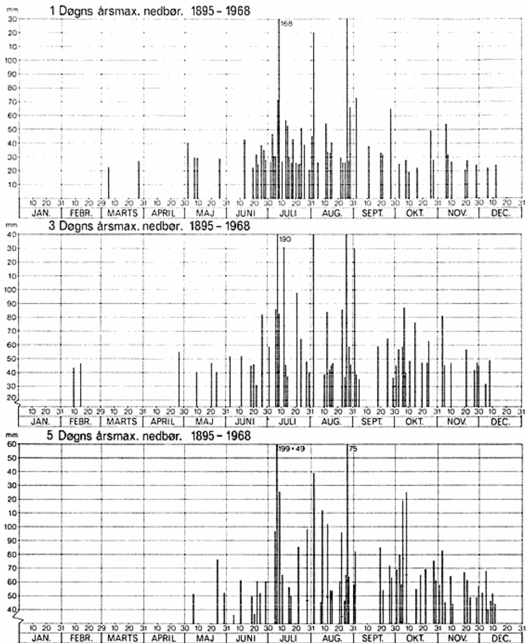
Fig. 9. Årsmaksima for 1-døgn, 3-døgn og 5-døgn, afsat på målingsdage; søjlehøjden angiver maksimas størrelse, en tværstreg at maksima er målt mere end én gang den pågældende dato.
