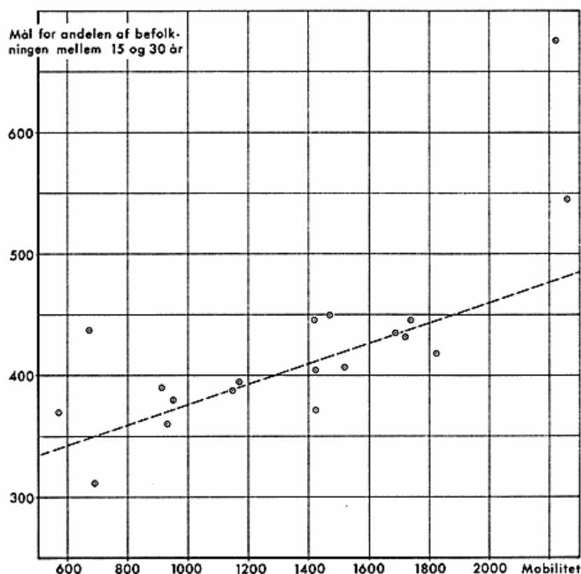
Fig. 13. Aldersstrukturens (ordinaten) betydning for kommunernes mobilitet (abscissen) 1961-65.
