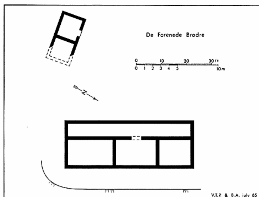
Fig. 13. Plan over plantagebygningen „De forenede Brødre“.
