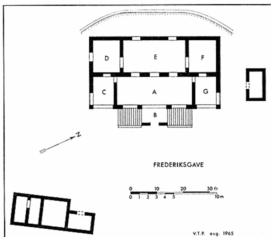
Fig. 9. Plan over plantagebygningen Frederiksgave.
