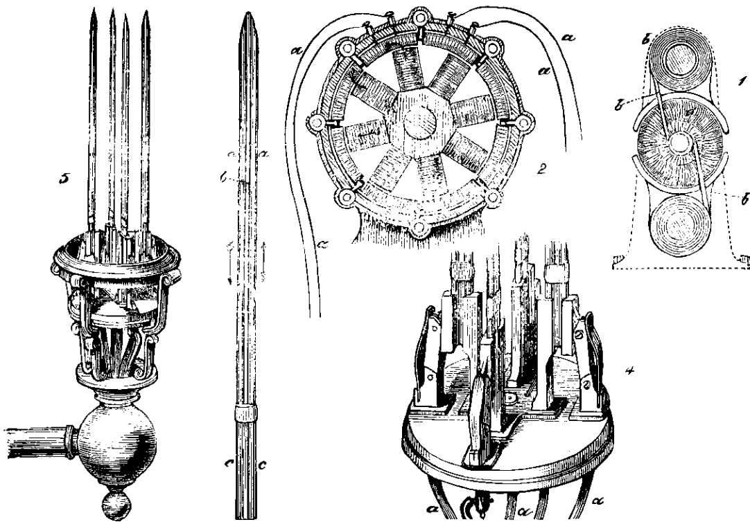
Jablochoffs elektriske Lysapparat.
