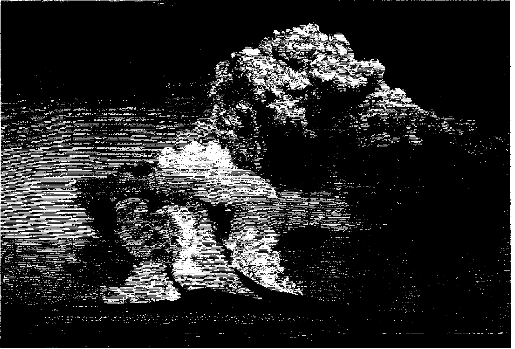
Vesuv under Udbrudet den 26de April 1872. Efter et Originalfotograf.
