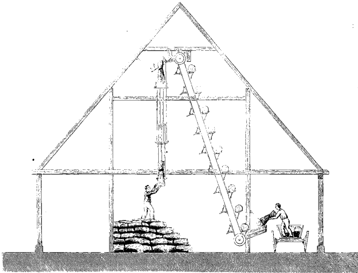
Gastrups Lademaskine.
