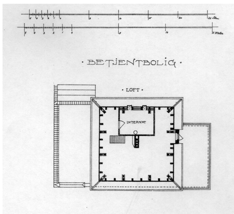
Arkitektens tegning fra 1907 af skolebetjentens loft med internatet.
